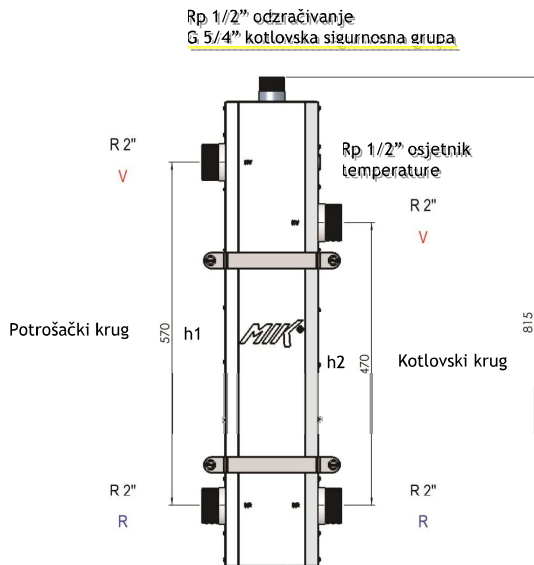
Rp 1/2" punjenje/praznjenje/ispiranje
