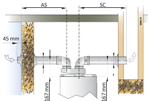
Primer sistema razdvojenih cevi (C 82 )
